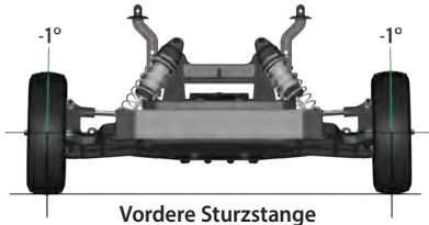
Vordere Sturzstange
